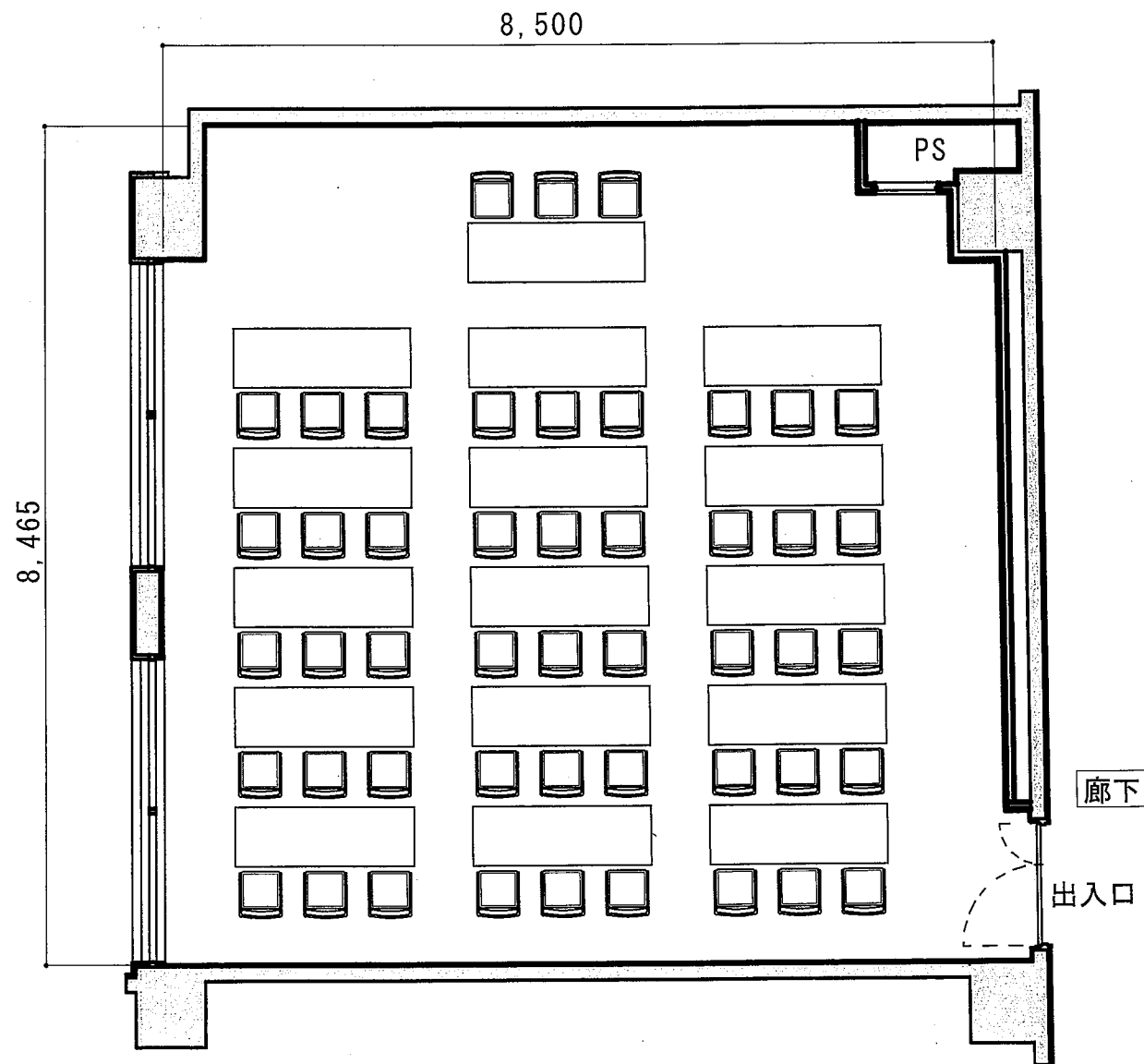
206号室配置図
